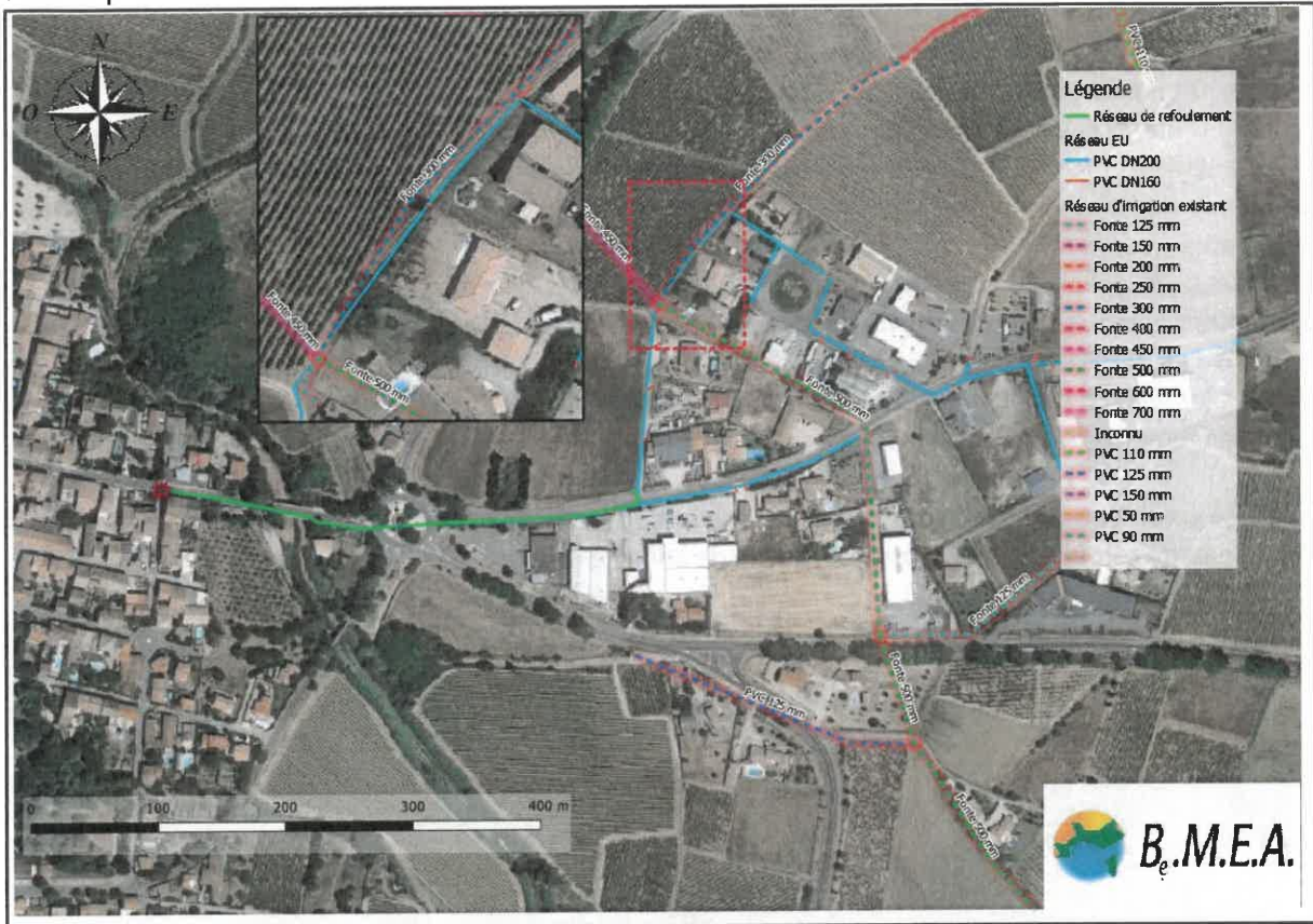
Pièce graphique n° 3 : Localisation du réseau d'irrigation existant
