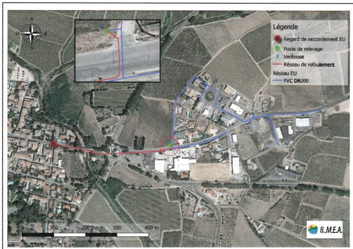
Pièce graphique n° 4 : Implantation générale du projet
